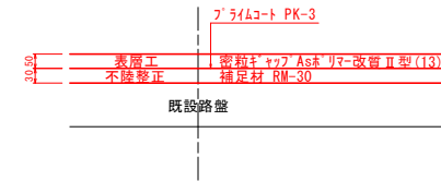
施工要領図
